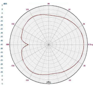
Fig. 2. Patrón cardiode
