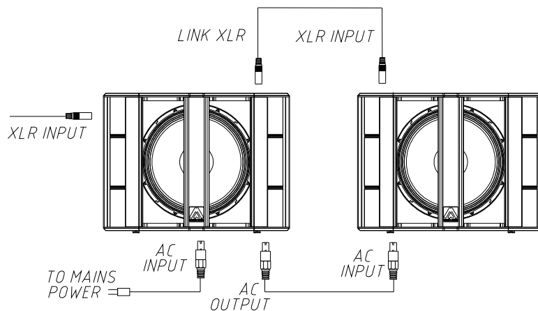
Fig. 8. Conexiones en paralelo para S18W
