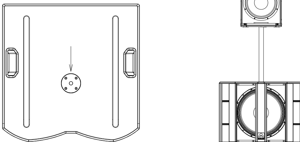
Fig. 9. Base para barra en S18W
