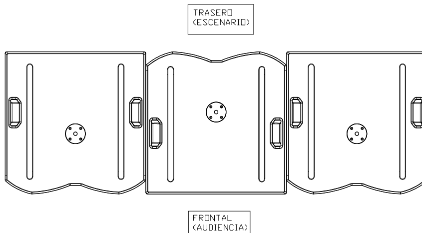
Fig. 4. Configuración cardiode básica para S18W (horizontal en suelo)
